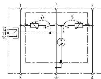
Prinzipschaltbild DR M 2P 30 FM
