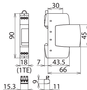
Maßbild DR M 2P 30 FM
