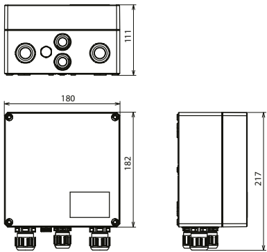
Maßbild DCU 2 YPV 1100 1M 2S
