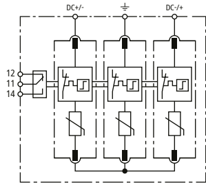
Prinzipschaltbild DCU 2 YPV 1100 1M 2S
