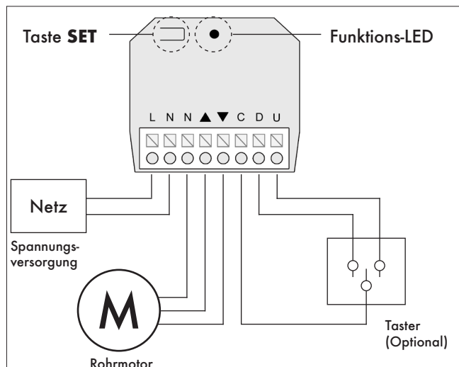
Abb.1: Anschlussplan Mercato Sotto
