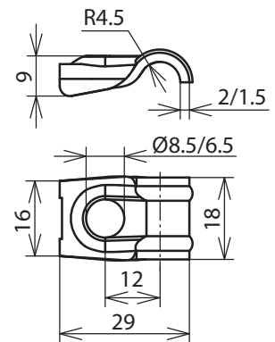
Maßbild UEL DQ 6.10 B8.5 V2A
