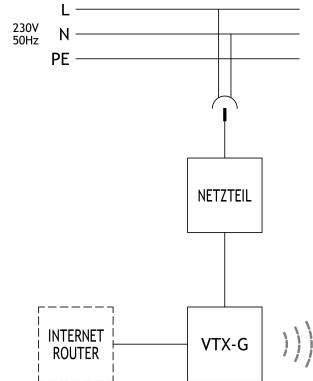
Abbildung 10: Schaltschema VTX-G
