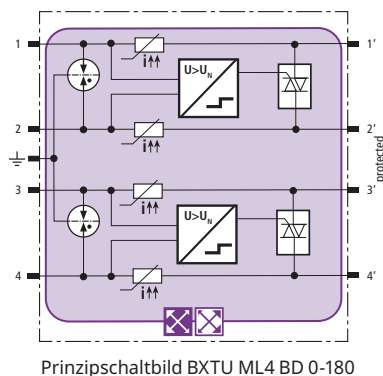
Prinzipschaltbild BXTU ML4 BD 0-180
