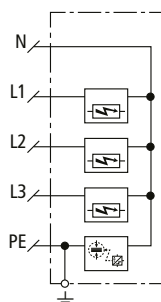
Prinzipschaltbild DSH ZP 2 TT 255
