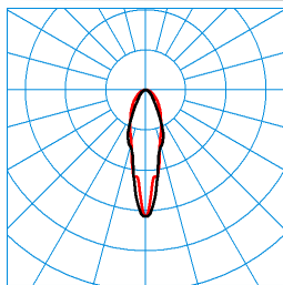
Cflex H1-E T 4000-840 UR I2 TX038385
