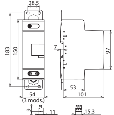
Maßbild DBM 1 CI 760 FM
