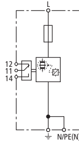
Prinzipialschaltbild DBM 1 CI 760 FM
