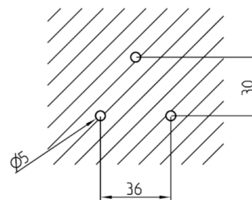
Bohrbild
