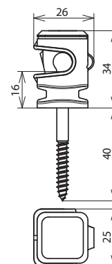
Maßbild LH DS 8 H16 HS5X50 GR
