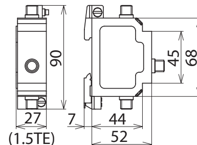
Maßbild DGA FF TV
