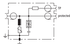
Prinzipschaltbild DGA FF TV
