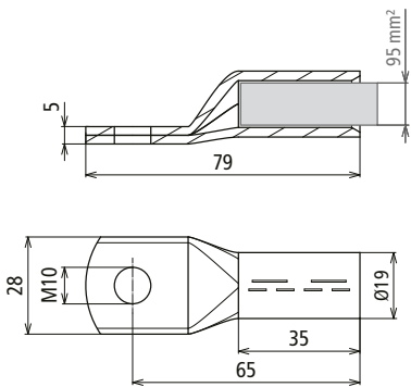
Maßbild PKS 95 10 CUGALNISN
