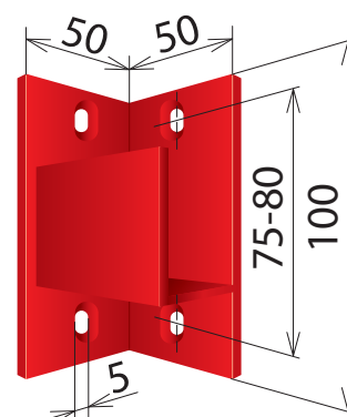
Maßbild H AB 32 46 K
