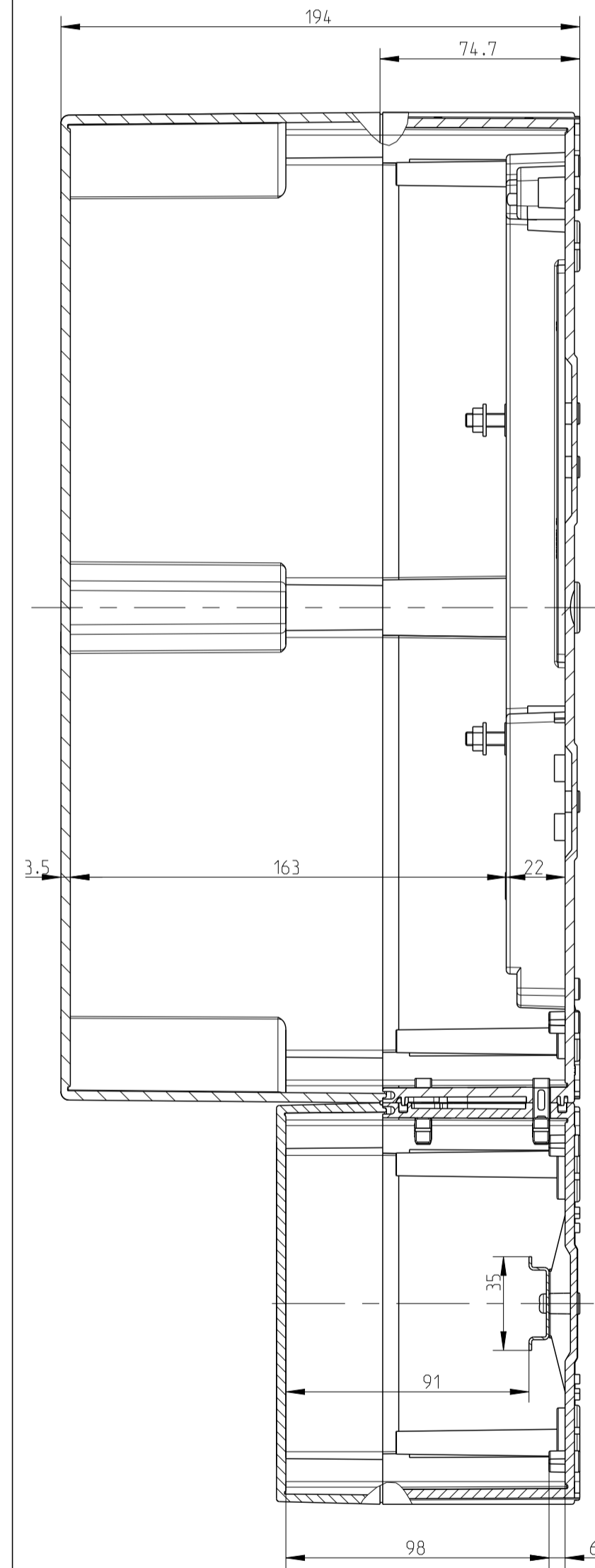
ZKi 100
