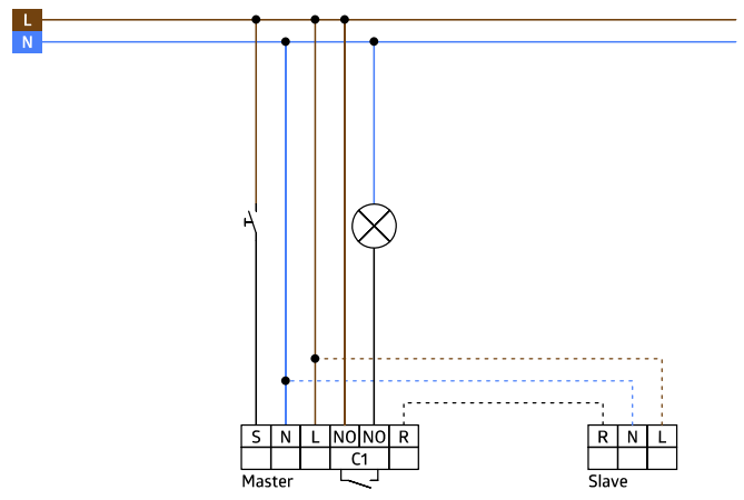
Schaltbild
