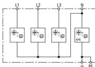
Prinzipschaltbild DSH TT 255
