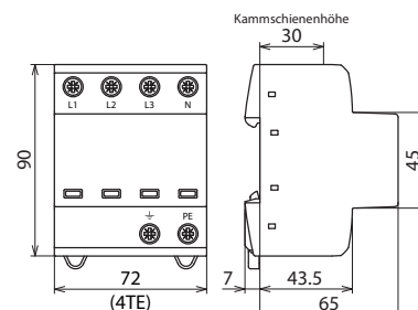
Maßbild DSH TT 255
