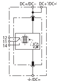
Prinzipialschaltbild DSE M 1 60 FM
