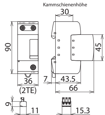
Maßbild DSE M 1 60 FM
