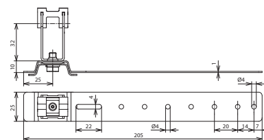
Maßbild DLH DG 8 H32 L205 V2A AL
