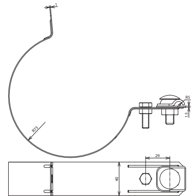
Maßbild ZMRRS 100 KB 6.10 CU STTZN
