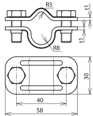
Maßbild UTK 8.10 16 STTZN
