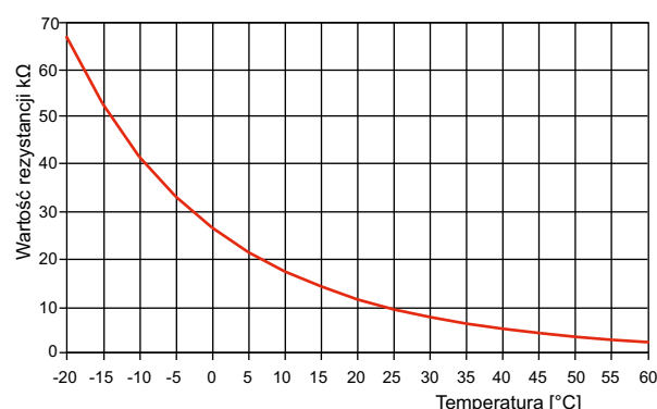
Rys. 7.3: Charakterystyka czujnika NTC-10
