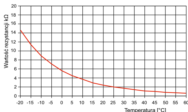
Rys. 7.4: Charakterystyka czujnika NTC-2 według DIN 44574 czujnik temperatury zewnętrznej
