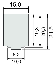
Ausschnittmaße
