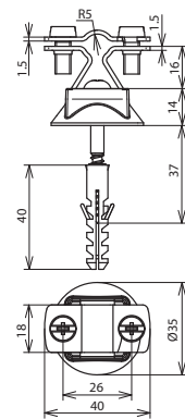
Maßbild LH ZS 8.10 FL20 KS KD8X40 V2A
