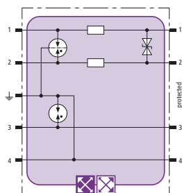
Prinzipschaltbild BXT ML2 BD S 48
