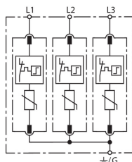
Prinzipialschaltbild DG MU 3PD 480 3W+G
