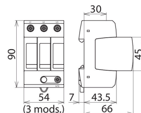
Maßbild DG MU 3PD 480 3W+G
