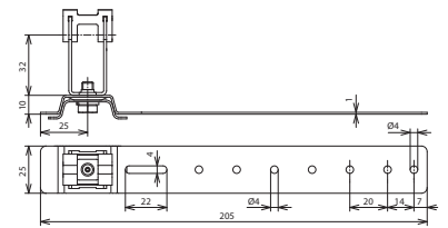
Maßbild
