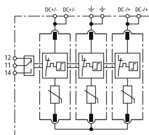
Prinzipschaltbild DCU 2 YPV 1100 1M 1S
