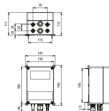
Maßbild DCU 2 YPV 1100 1M 1S MC4 FM
