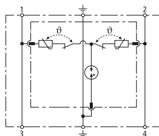
Prinzipschaltbild DR M 2P 30
