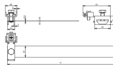
Maßbild BRS 27.168 AQ4 25 V2A
