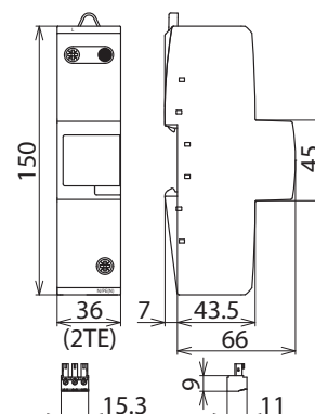
Maßbild DVCI 1 255 FM
