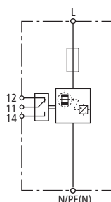
Prinzipialschaltbild DVCI 1 255 FM
