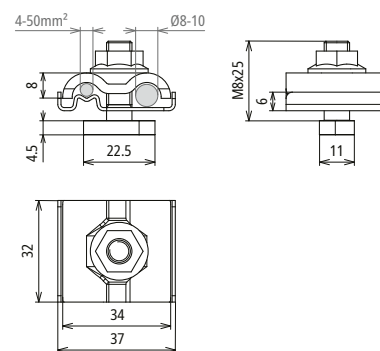
Maßbild UEK 8.10 AQ4 50 HKSM8X25 V2A
