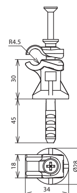
Maßbild LH DFI DQ 6.10 V2A H30 GR
