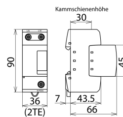
Maßbild DBH M 1 255
