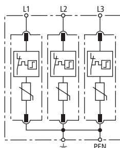
Prinzip Schaltbild DG M TNC 275
