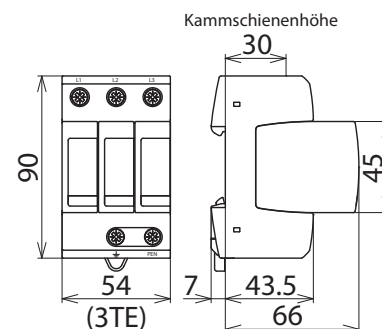
Maßbild DG M TNC 275
