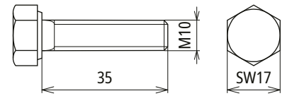
Maßbild SKS M10X35 DIN 933 V2A
