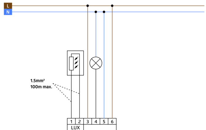
Schaltbild
