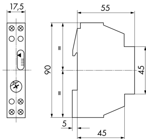
Bemaßung 92681
