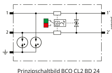
Prinzipschaltbild BCO CL2 BD 24
