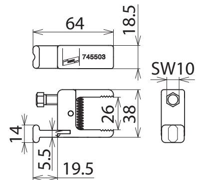
Maßbild KK TA 0 24 SK10
