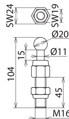
Maßbild KFP 20 M16 45 SSM
