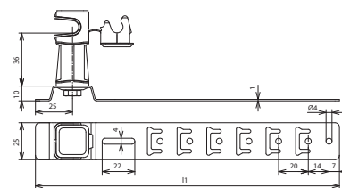
Maßbild DLH US 8 H36 L335 GR V2A
