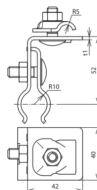
Maßbild DLH KB 6.10 RSF20.25 V2A
