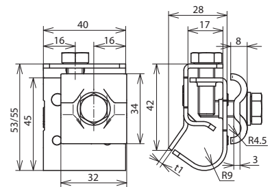
Maßbild DRK DUL 8.10 W16.22 STTZN
