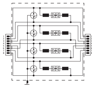
Prinzipschaltbild DPA M CAT6 RJ45S 48
