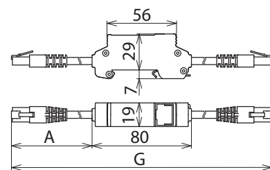
Maßbild DPA M CAT6 RJ45S 48
