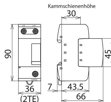
Maßbild DB M 1 255
