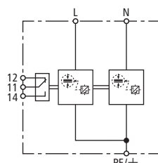
Prinzipschaltbild DSH TN 255 FM
