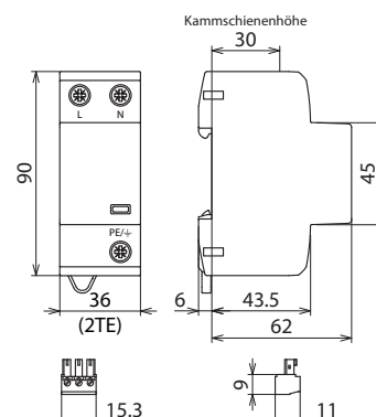
Maßbild DSH TN 255 FM
