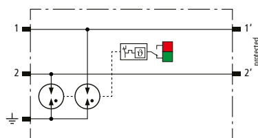
Prinzipschaltbild BCO MOD ML2 B 180
