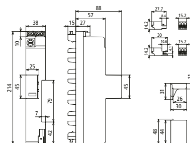
Maßbild DSH ZP 2 SG TNC 255
