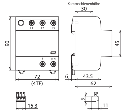
Maßbild DSH TNC 255 FM
