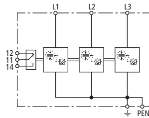
Prinzipschaltbild DSH TNC 255 FM
