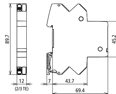
Maßbild BCO CL2 BD HC10A 24
